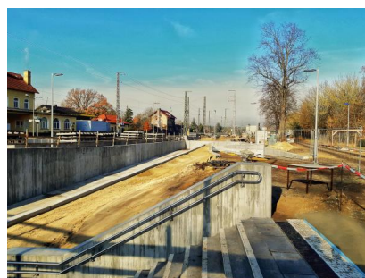
Die Personenunterführung im Bahnhof Wünsdorf-Waldstadt wurde im November 2021 eröffnet. Die Rampe an der Westseite wird bis April 2022 fertiggestellt. Bis dahin gibt es einen bauzeitlichen Aufzug für die barrierefreie Querung der Gleise (November 2021) [Quelle: DB Netz AG]
