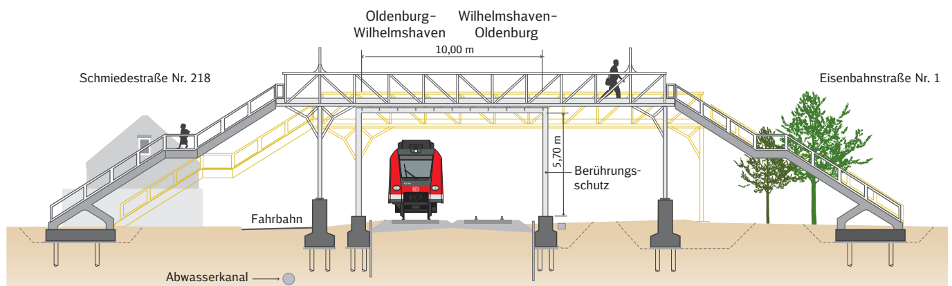
Vergleich: Die Fußgängerüberführung Bant vor und nach dem Anheben des Bauwerks.
