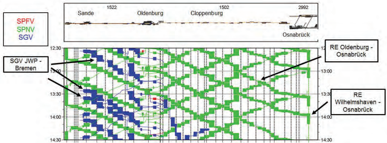
Abbildung 10: Ausschnitt Bildfahrplan (12:30-14:30 Uhr) Wilhelmshaven – Oldenburg – Osnabrück für den Zielzustand
