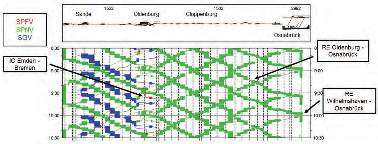
Abbildung 9: Ausschnitt Bildfahrplan (08:30-10:30 Uhr) Wilhelmshaven – Oldenburg – Osnabrück für den Zielzustand
